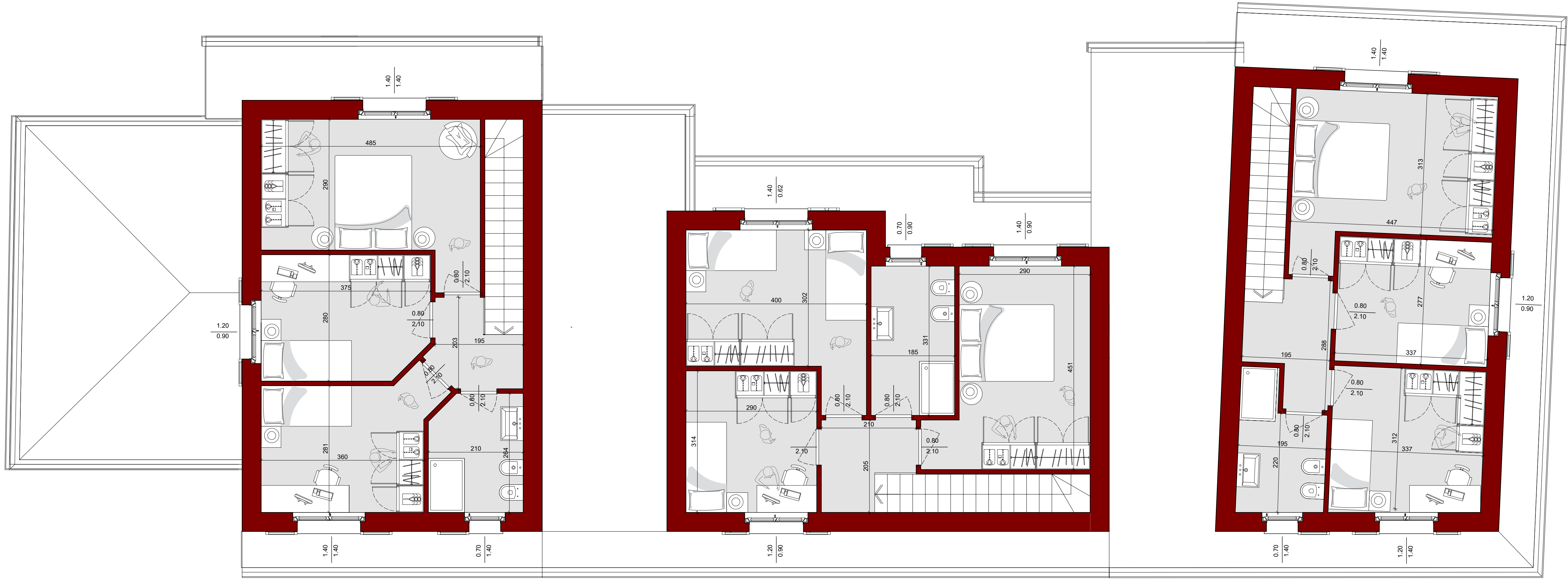
PIANTA PIANO SOTTOTETTO
